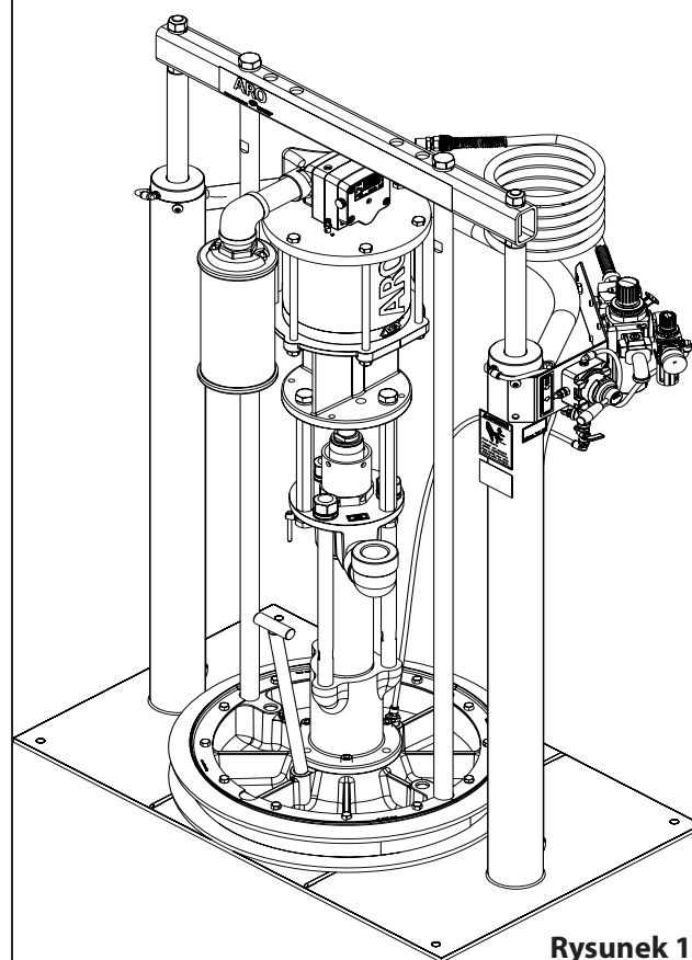
TP0813S5XXXXXXX ZESPÓŁ TŁOKA
