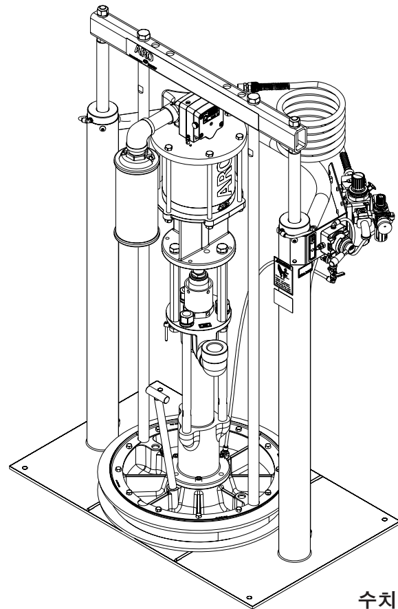
TP0813S5XXXXXXX 램 패키지
