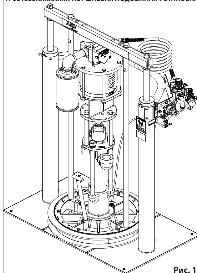
ТР0813S5XXXXXXX ПОРШНЕВАЯ ПОДЪЕМНАЯ УСТАНОВКА
